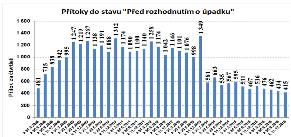
Obr.č. 20: Čtvrtletní přítoky ins.návrhů do stavu „Před rozh. o úpadku“
