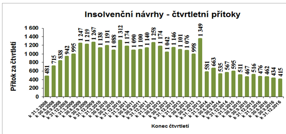
Obr.č. 2: Přítoky insolvenčních návrhů do systému (externí vstup)
