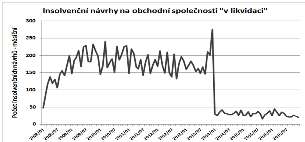
Obr.č. 14: Přítoky ins. návrhů na obch. společnosti „v likvidaci“
