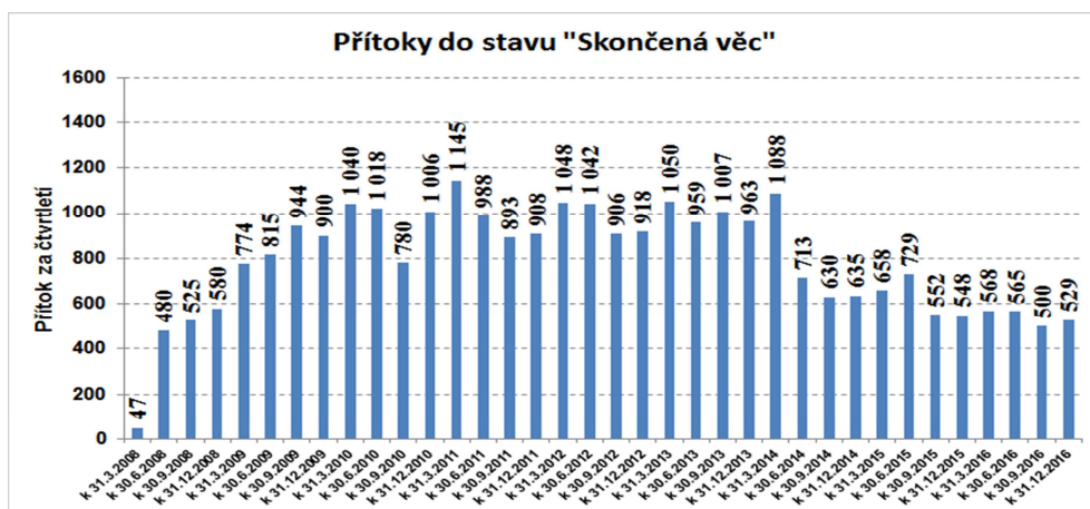
Obr.č. 48: Přítoky insolvenčních řízení do stavu „Skončená věc“
