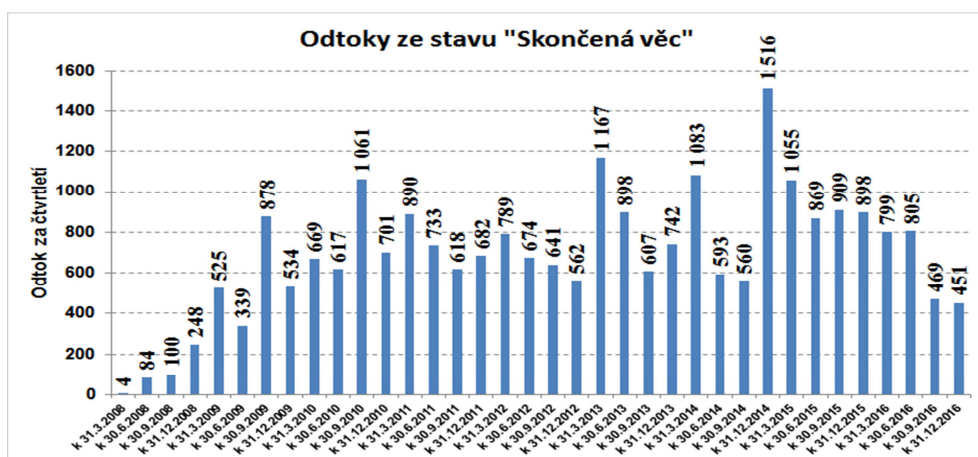
Obr.č. 49: Odtoky insolvenčních řízení ze stavu „Skončená věc“
